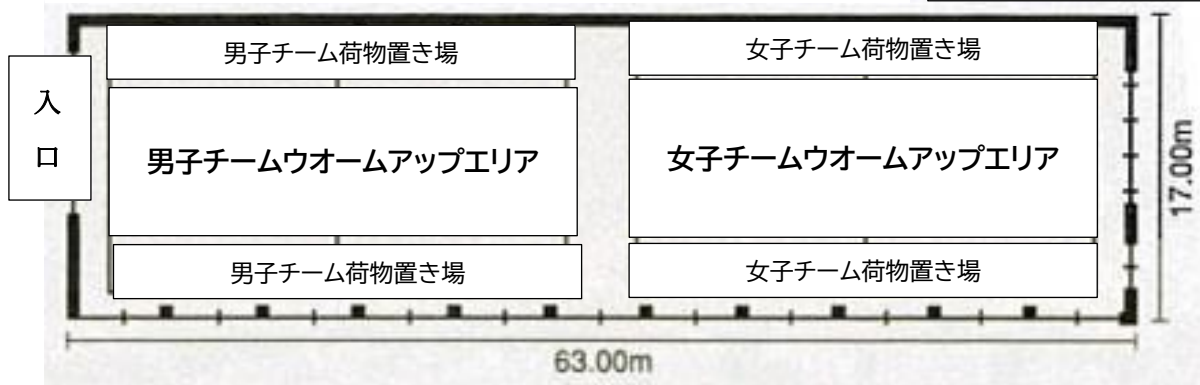
荷物置き場・アップフロア(1階)平面図
